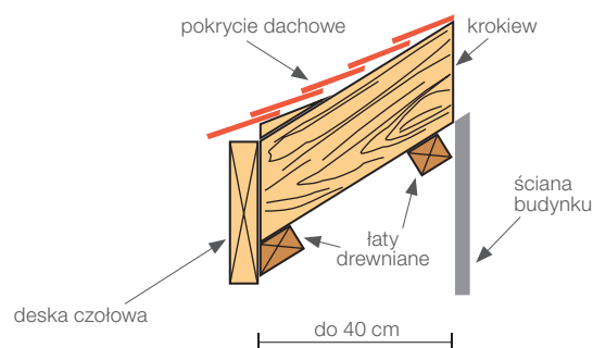
wysunięcie okapu do 40 cm
